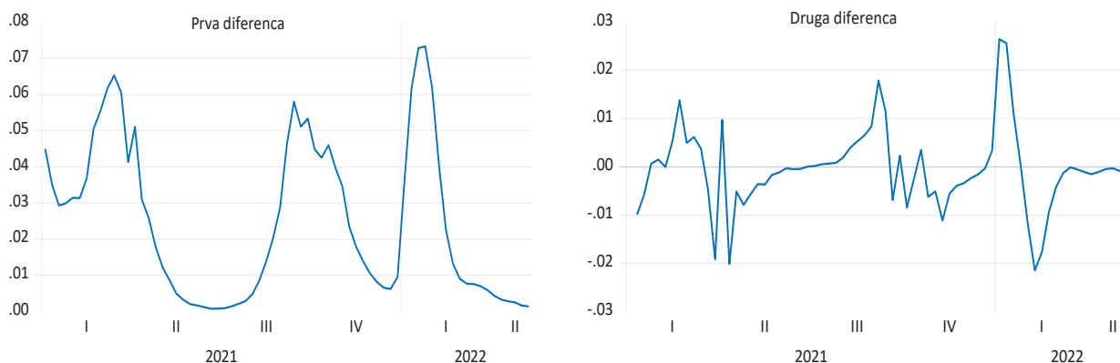
Grafik 1: Polazna serija, prva i druga diferencija polazne serije
