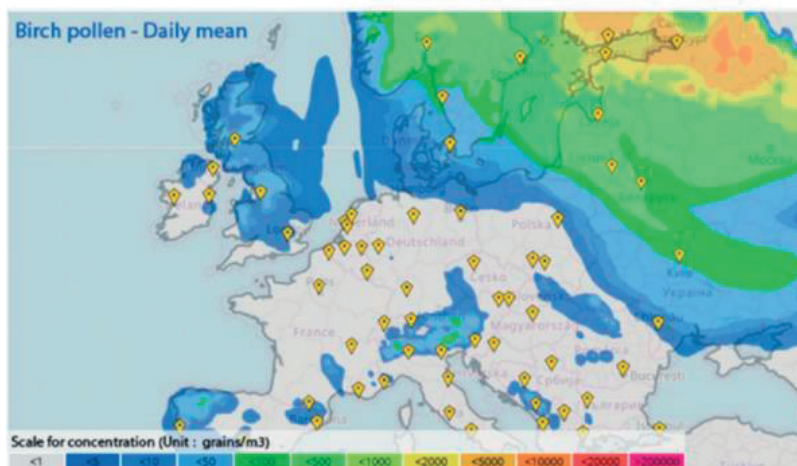
Slika 2: Koncentracija polena na području Evrope [3]
