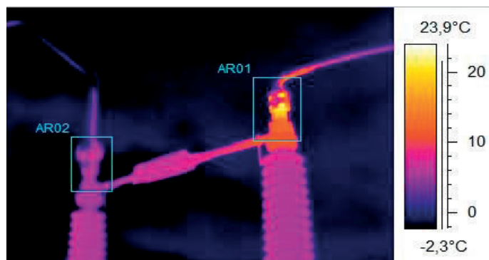
Slika 7: Termogram linijskog rastavljača [3]
