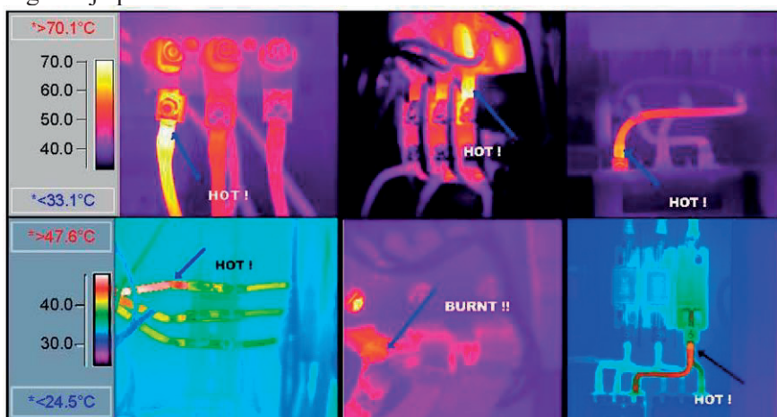
Slika 1: Primjena termografije u energetici [5]
