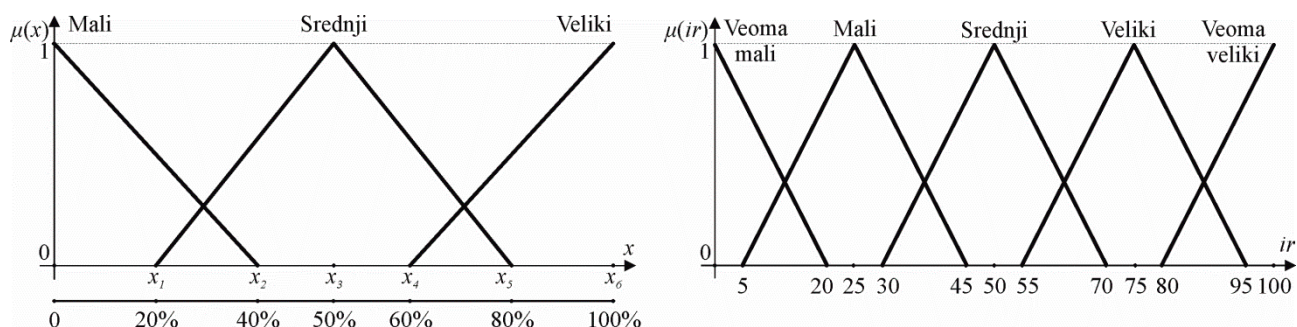
Slika 2: Funkcije pripadnosti fazi skupova X_M , X_S , X_V , IR_{VM} , IR_M , IR_S , IR_V i IR_{VV}
