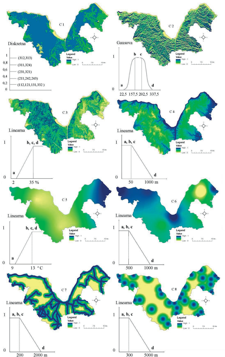
Slika 1: Standardizovani kriterijumi sa oblikom fuzzy članstva
